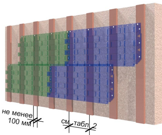
Рис. 3 Вертикальная обрешётка под фасадные панели Döcke ФЛЕМИШ, KLINKER, STERN, СЛАНЕЦ, ДЮФУР
