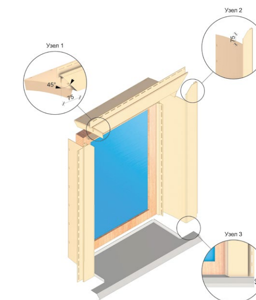
Рис. 18 Обрамление оконного проёма при помощи околооконного профиля 75/200/13 мм (только для ЭДЕЛЬ) при наличии металлического отлива.
