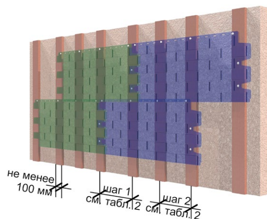
Рис. 4 Вертикальная обрешётка под фасадные панели Döcke BERG
